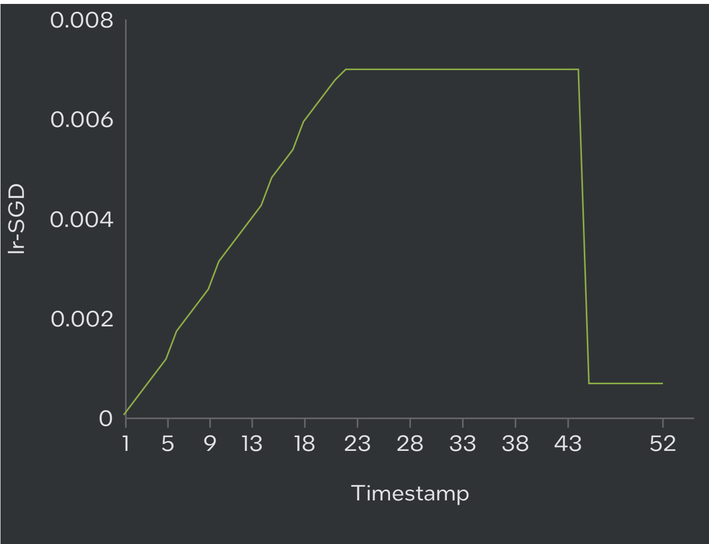
lr-SGD
