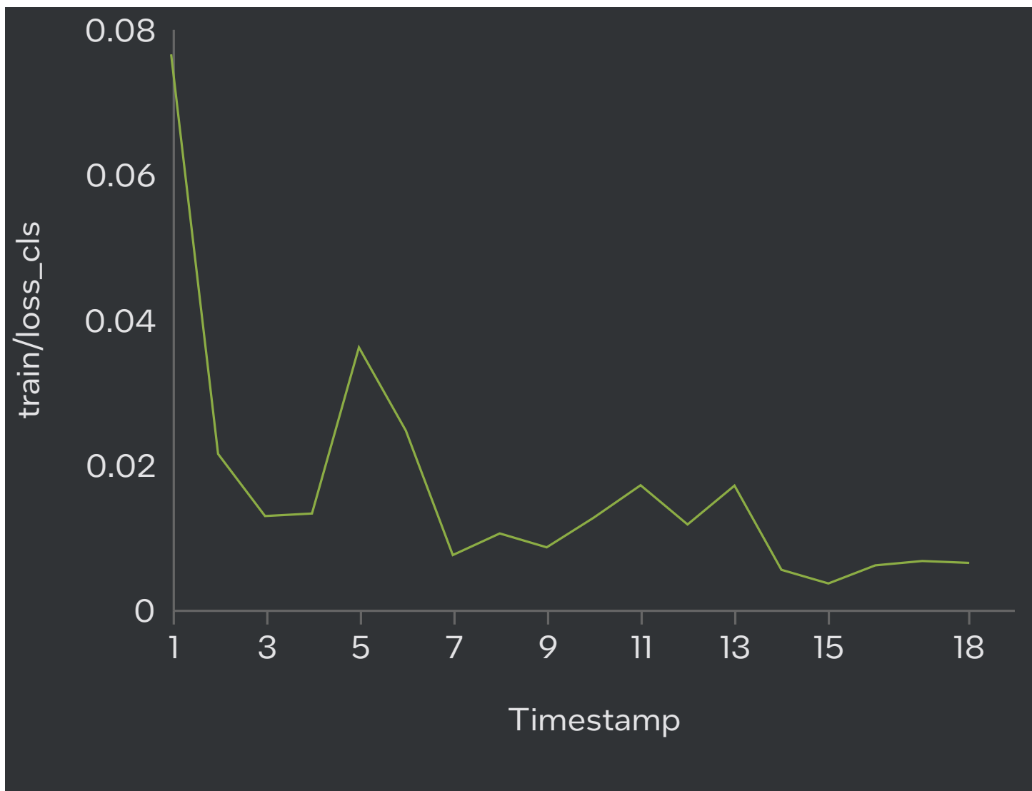
train/loss_cls
