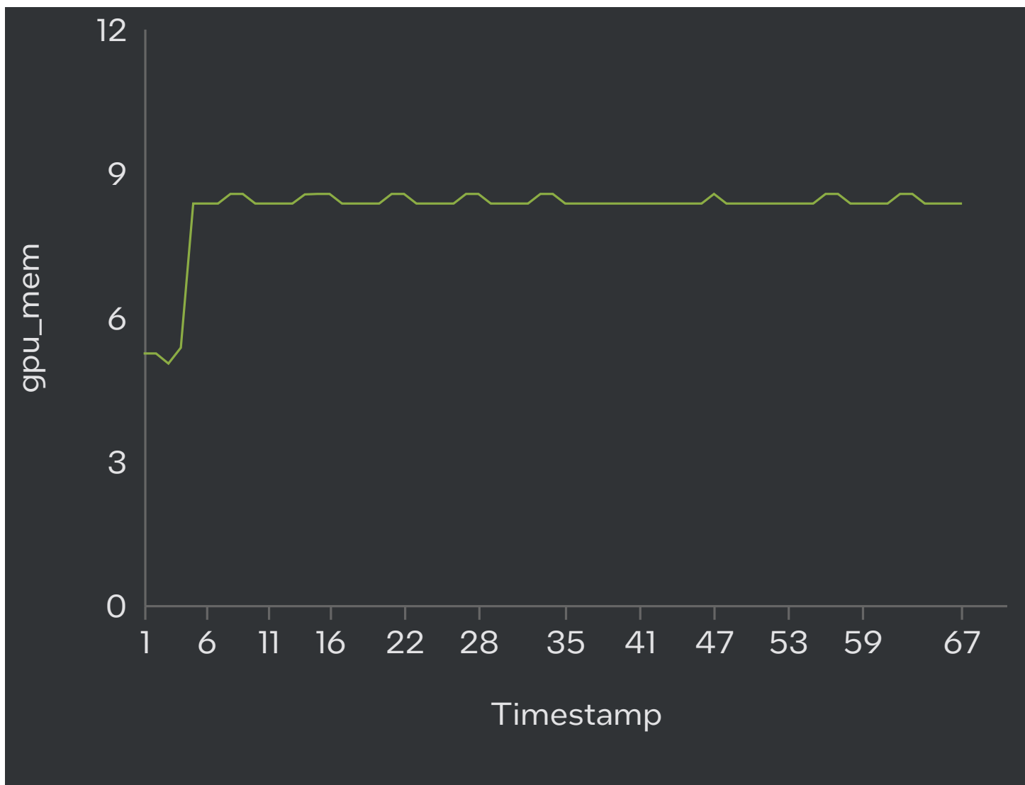
gpu_mem
