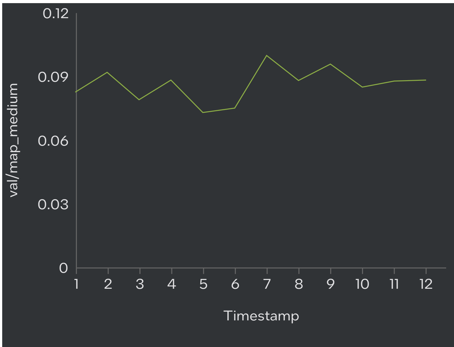
val/map_medium
