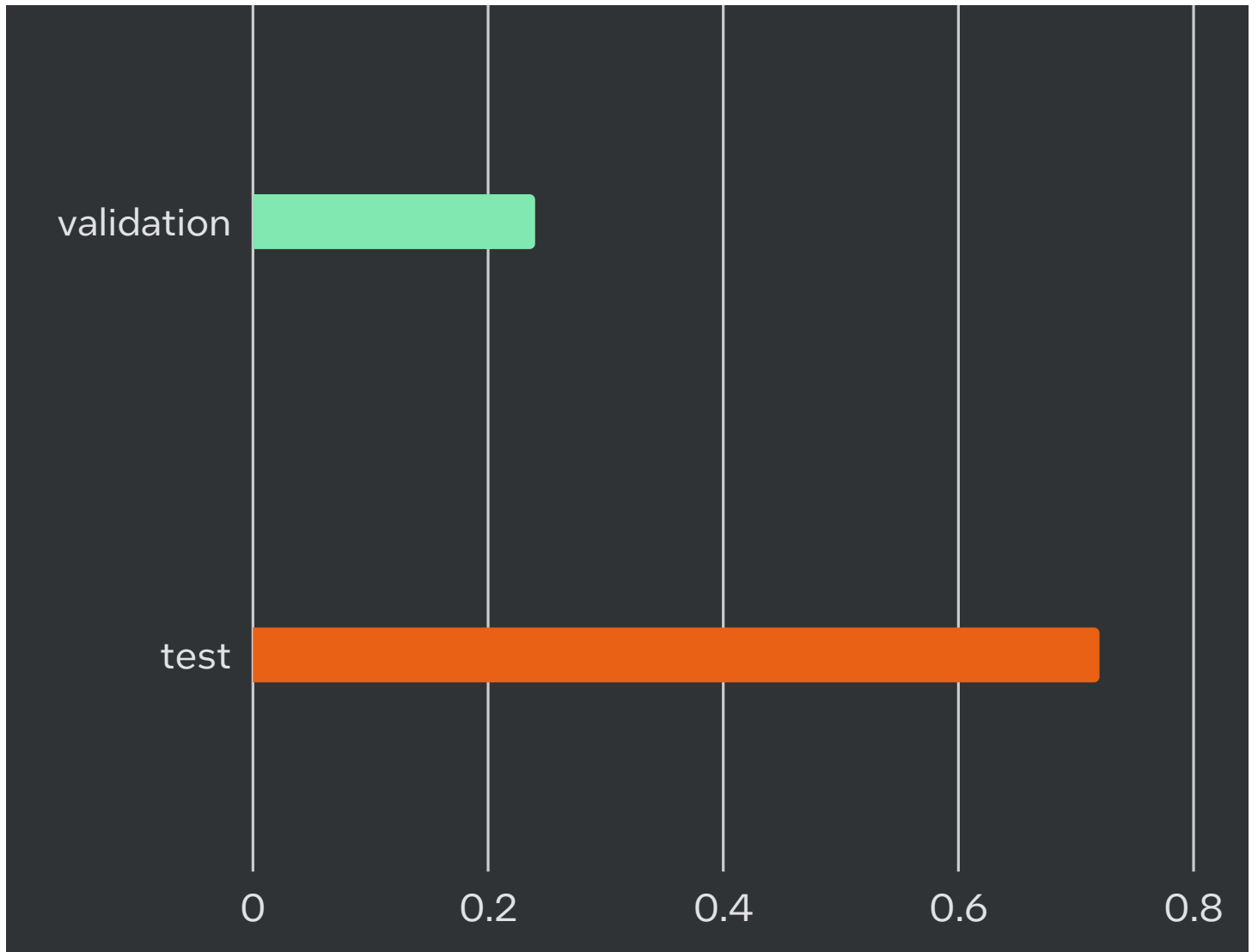
Dice
