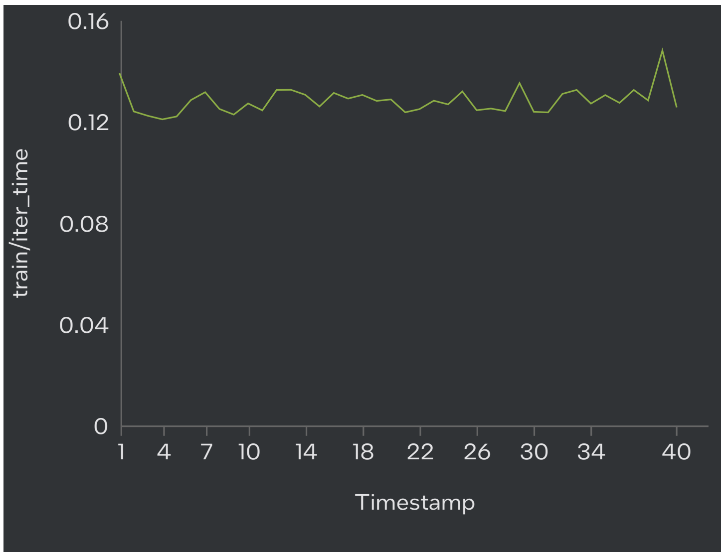
train/iter_time
