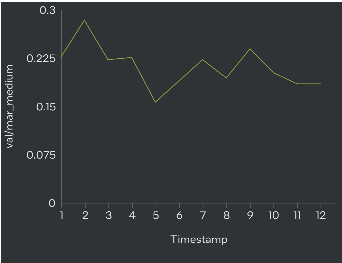
val/mar_medium
