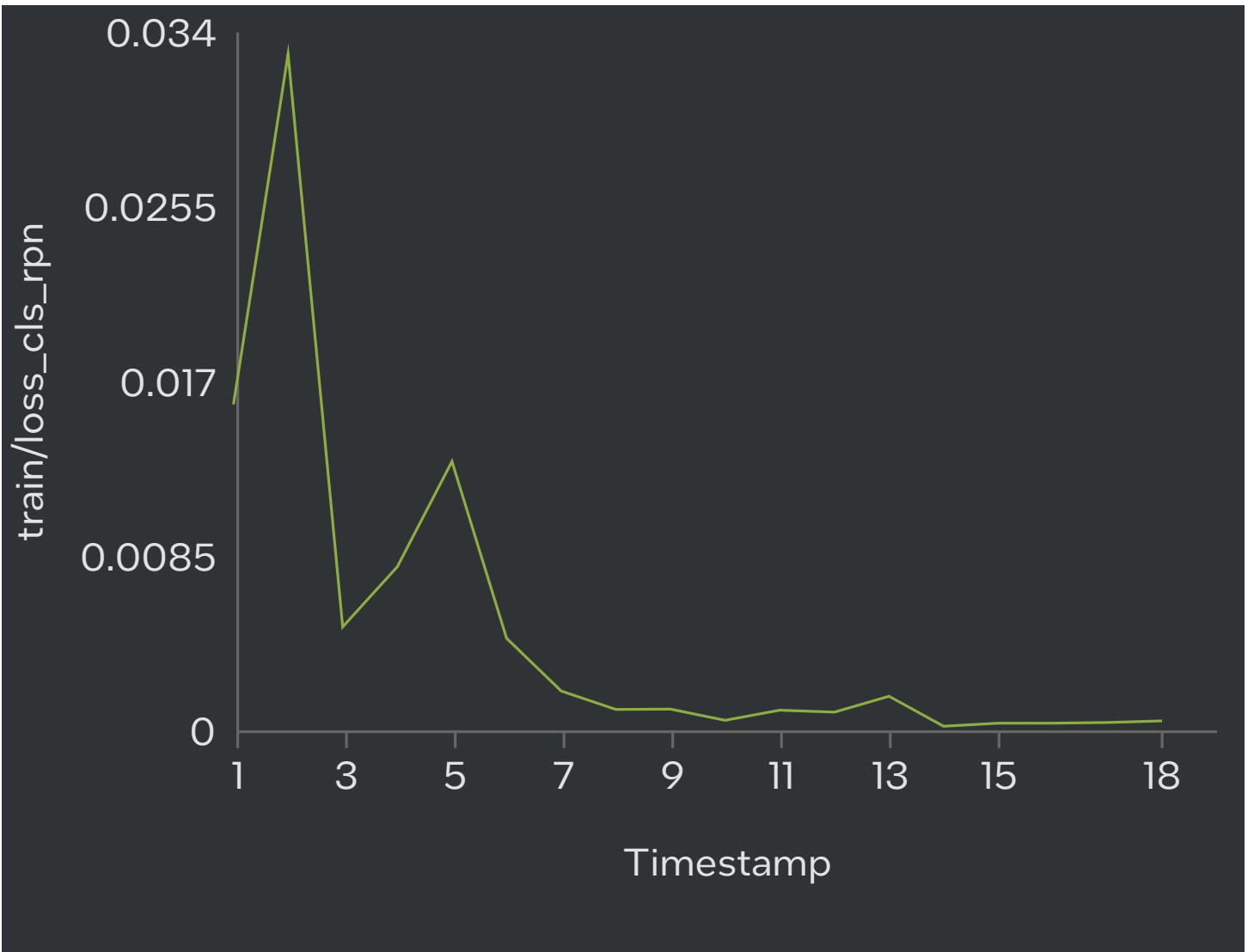
train/loss_cls_rpn
